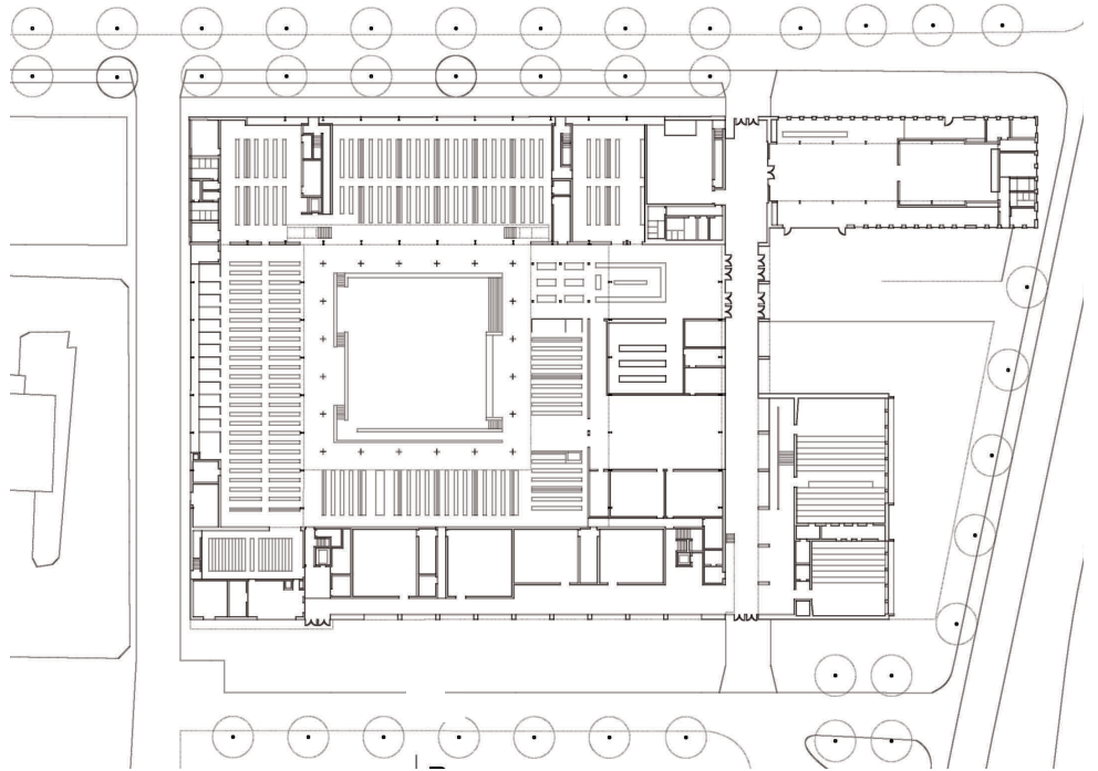
ERDGESCHOSS
